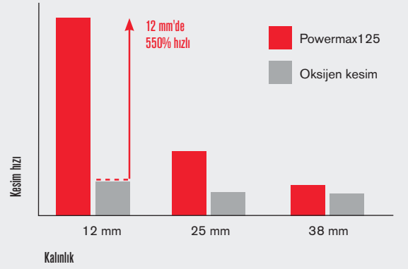
Yumuşak çelikte kesme hızları karşılaştırması
